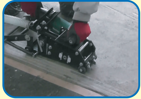
エポキシ樹脂モルタル5mm厚
